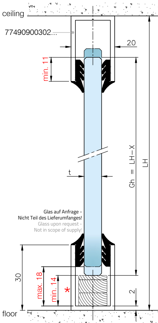
Aufmaß mit U-Profil 30x20x30: Site measuring with U-profile 30x20x30:
