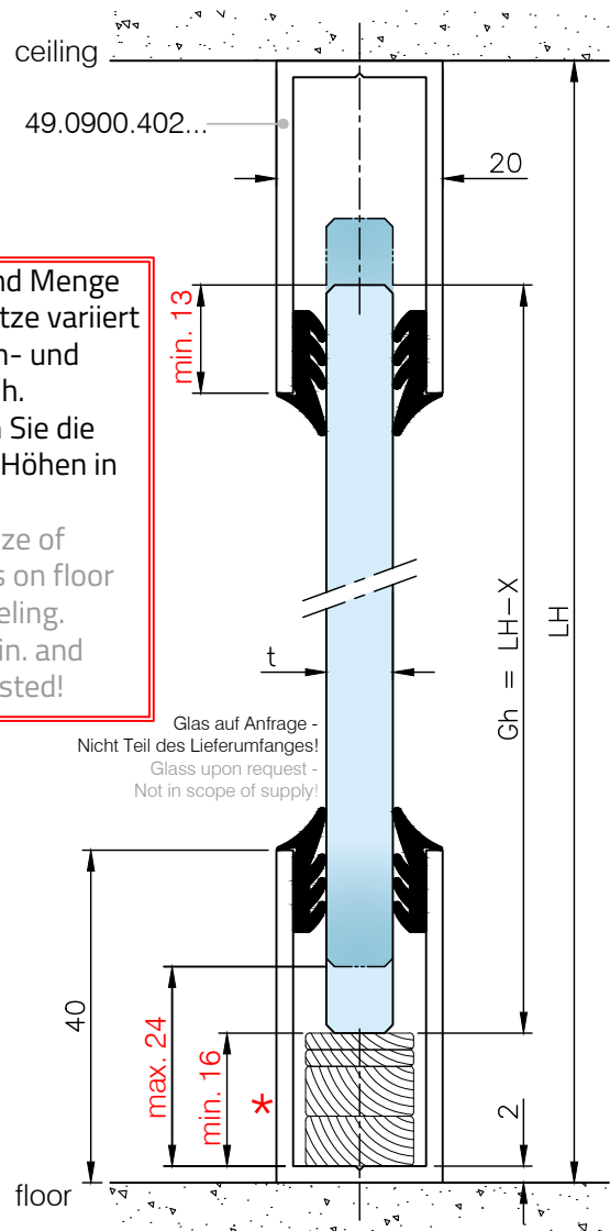
Aufmaß mit U-Profil 40x20x40: Site measuring with U-profile 40x20x40:
