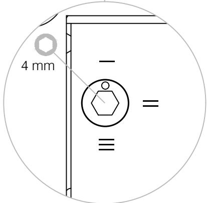
Einstellung der Kraft: power adjustment:
